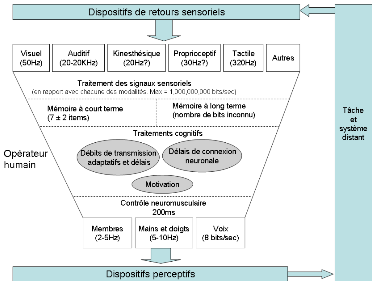
FIGURE 2.20 – Asymétrie des besoins fréquentiels dans le traitement de l'information haptique. D'après Brooks (1990).
