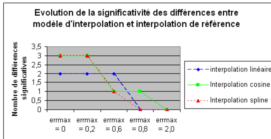
FIGURE 4.9 – Evolution du nombre de différences significatives entre les modèles d’interpolation, en fonction de l’interpolation de référence et de l’amplitude du bruit Err_{max} utilisé. Chaque point de la courbe représente le nombre de différences significatives de la figure 4.8 obtenue précédemment. On observe donc une diminution de l’influence du modèle d’interpolation avec l’accroissement de l’erreur.
