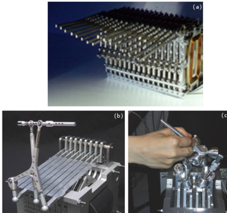
FIGURE 2.17 – Clavier rétroactif modulaire (Cadoz 1990). a) configuration de base 18 touches. b) configuration simulant un dispositif spécifique. c) configuration joystick à 6 degrés de liberté.
