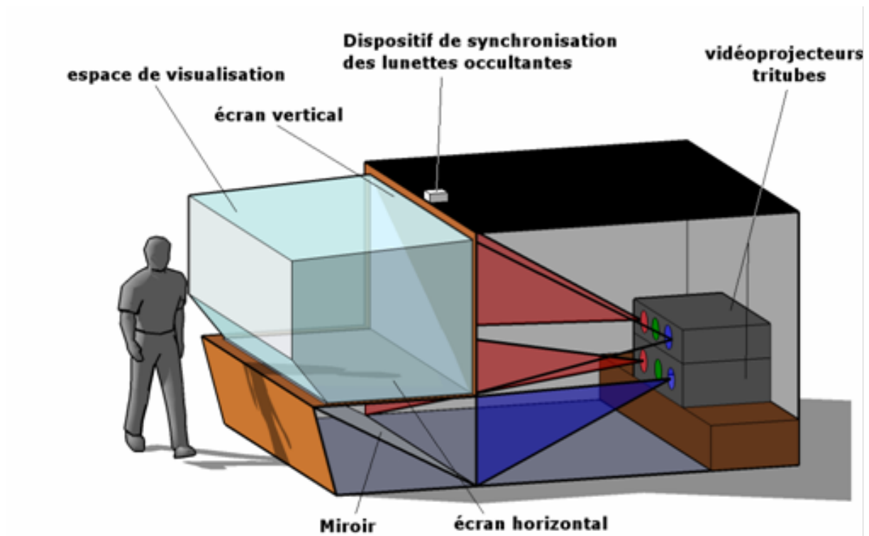
FIGURE 7.8 – Vue éclatée du workbench. Pour la description des différents éléments, voir le texte.
