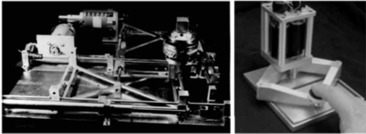
FIGURE 2.15 – a). Dispositif à retour d'effort planaire de haute puissance (Ellis 1996). b) Pantograph. Dispositif pour simuler l'exploration de surfaces (Ramstein 1994)
