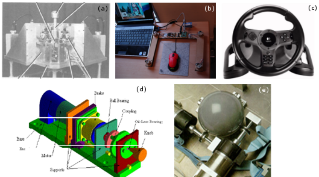
FIGURE 2.14 – (de haut en bas, de gauche à droite). a). Joystick à retour d'effort d'après (Adelstein 1990). b). Souris à retour d'effort à base de câble (Ishiii 2009). c). Volant à retour d'effort (Logitech 2009). d). Contrôleur rotatif à retour d'effort (Badescu 2002). e). Trackball à retour d'effort (d'après J.F. Schouten School)
