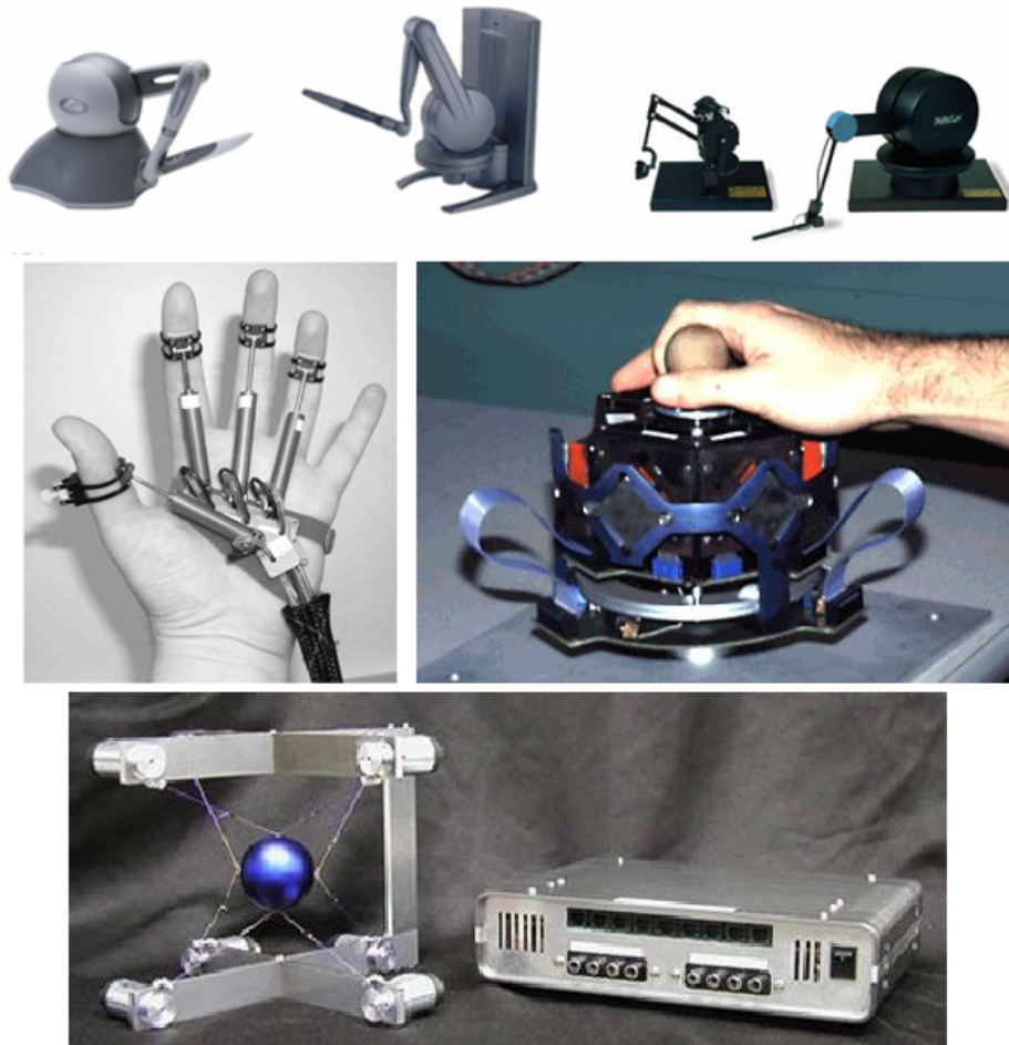
FIGURE 2.16 – a) Gammes des dispositifs à retour d’effort de SensAble (Phantom Omni, Phantom Desktop, Phantom Premium 1.0 et 1.5) (Salisbury 1995). b) Gant à retour d’effort (Master II-ND) à base de pistons pneumatiques (Burdea 1992). c) Magnetic Levitation Haptic Device (Berkelman 1995). d) Système à retour d’effort à base de câble et son contrôleur (SPIDAR-G)(Sato 1992).
