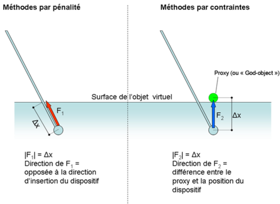
FIGURE 2.21 – Principales méthodes de rendu haptique
