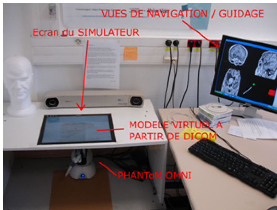
FIGURE 8.11 – Prototype de simulateur chirurgical en base du crâne développé. Le retour d'effort est assuré par le dispositif haptique (Phantom Omni), situé sous l'écran de visualisation placé horizontalement. Une localisation de la position du dispositif haptique dans les données anatomique est possible sur un écran déporté.
